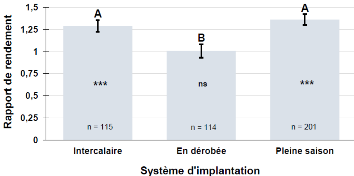
Figure 4.8 Effet du système d'implantation des CC sur le rendement des céréales
